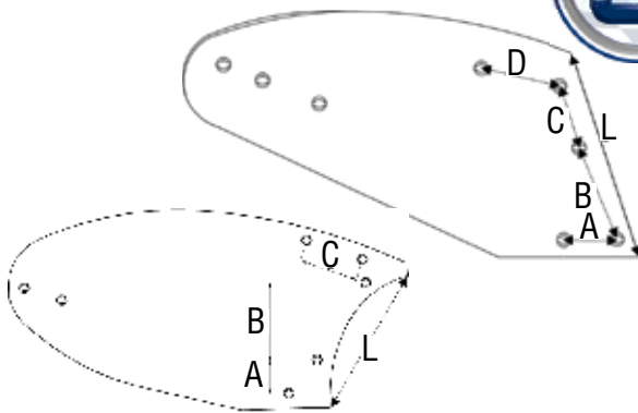
Streichblech-Hinterteil
