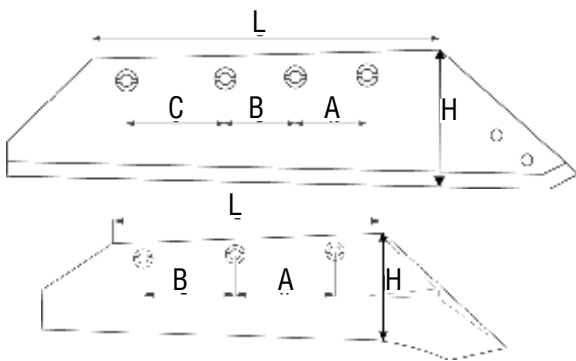
Schnabelschar - Wechselspitzschar
