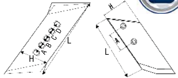
Düngereinleger - D-Riester
